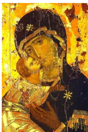
Рис. 2. Богоматерь. Ситуация, обозначаемая числом \text{ДВА}=\text{До}+\text{УА} .
